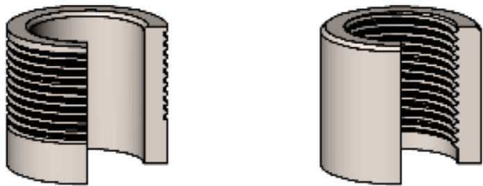
Рис.8 - Резьбовые соединения
