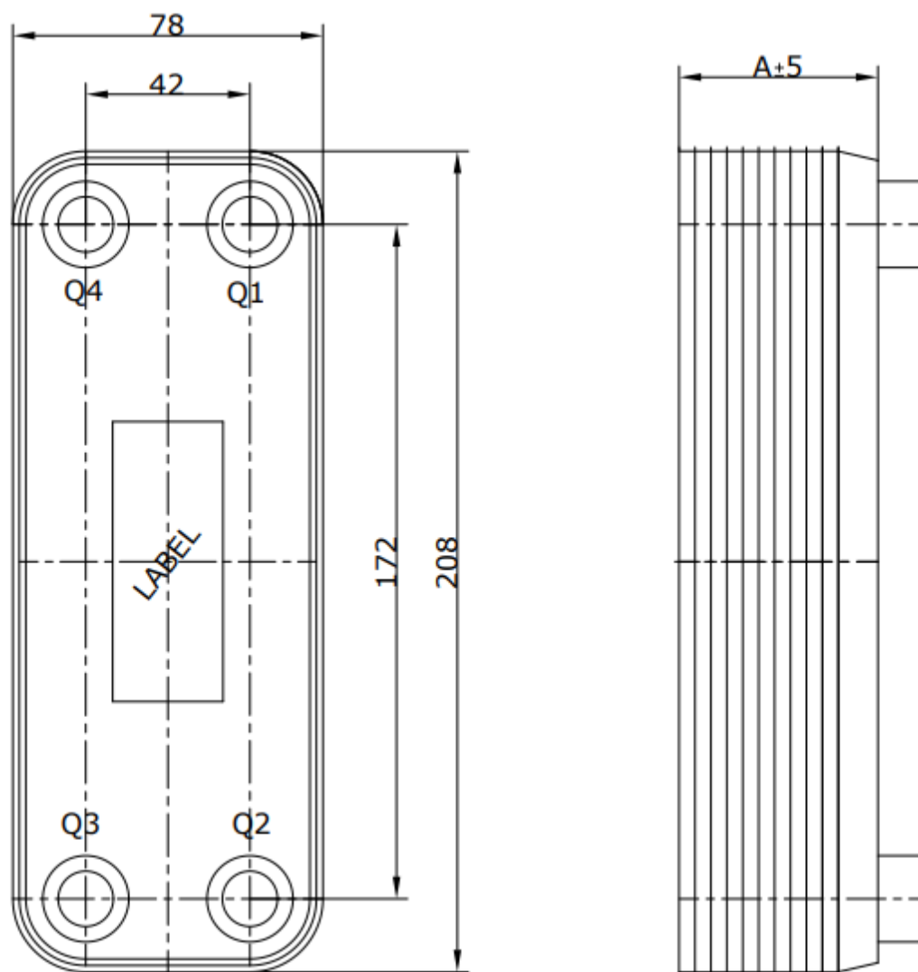
Рис.6 - Габаритные размеры и изображение теплообменника пластинчатого модификации BPHE_RD-014W
