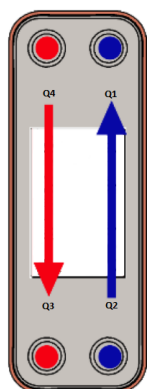
Рис.11 – Направление потоков
