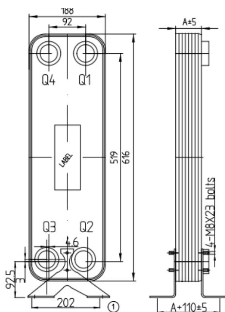
Рис.6 - Габаритные размеры и изображение теплообменника пластинчатого модификации BPHE_RD-095
