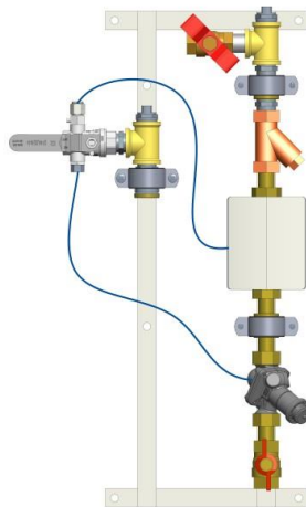
Рис. 1. Общий вид изделия ШКСО-1Р тип 5 с комбинированным клапаном APQT
