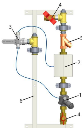
Рис. 2. Состав ШКСО-1Р тип 5
